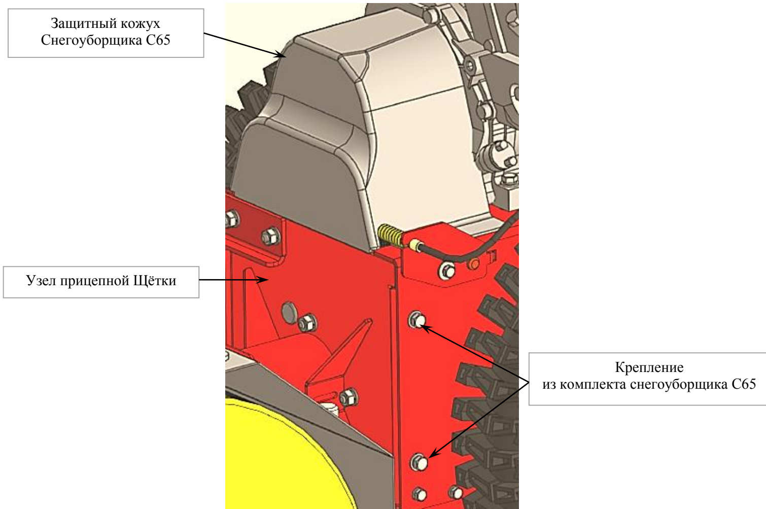
РИС.3 СХЕМА ЗАКРЕПЛЕНИЯ ЩЁТКИ НА СНЕГОУБОРЩИКЕ С65.
